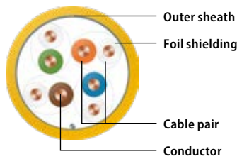
F/UTP
