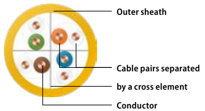
U/UTP
